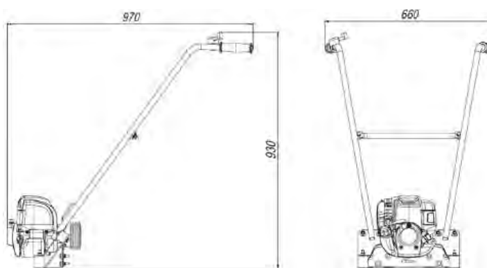
Рис. 1. Габаритные размеры виброузла
