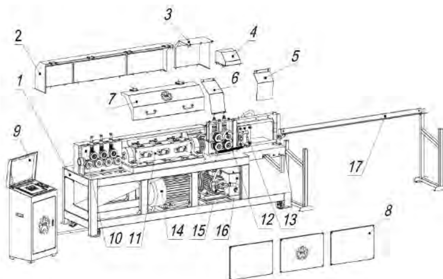
Рис. 1. Схема устройства правильно-отрезного станка VKP ПРО-16:
